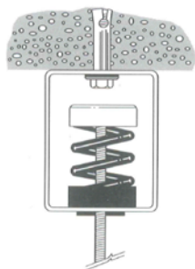
Montaje con contacto directo
